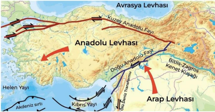
Resim 58: Arap levhası Anadolu levhasını batıya doğru itmektedir
