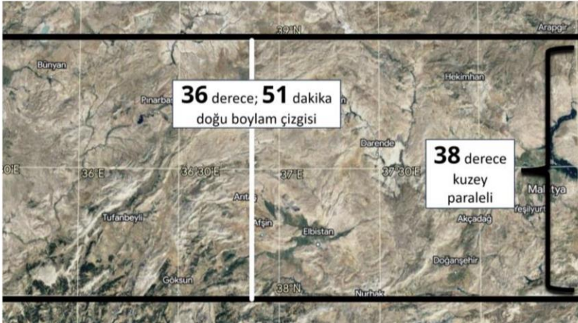
Resim 55: 38 derece kuzey enleminde 36 derece 51 dakika doğu boylamına sahip olan yerler beyaz çizgiyle çizilmiştir.
